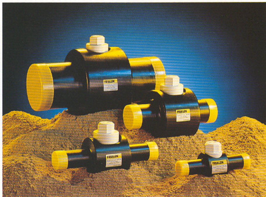
Шаровой вентиль ФРИАЛЕН® для газопроводов. 1/4 оборота и магистраль перекрыта.
